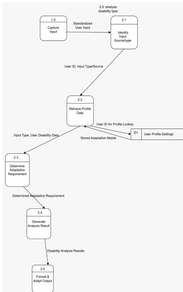
2.2.2.3 DFD (Level 2)
