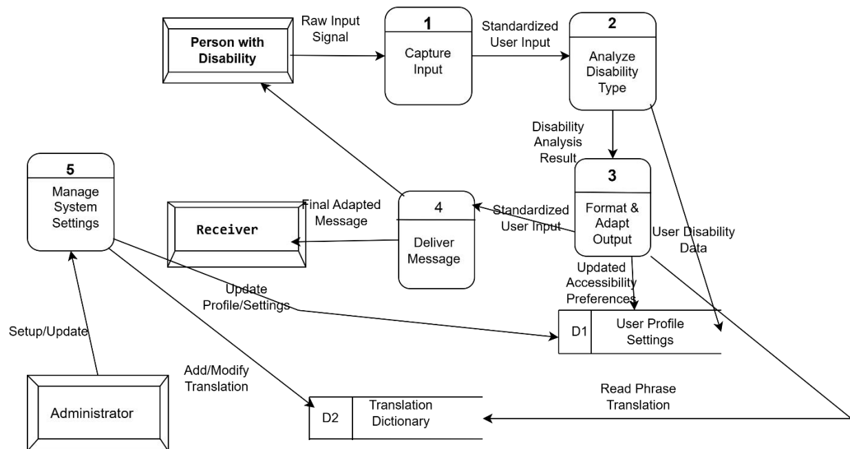
2.2.2.3 DFD (Level 2)
